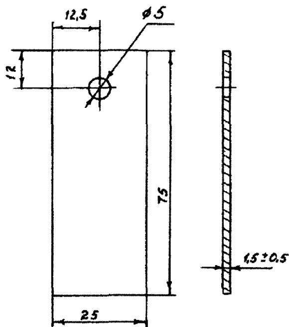
Рисунок 2. Эталонная металлическая пластина
