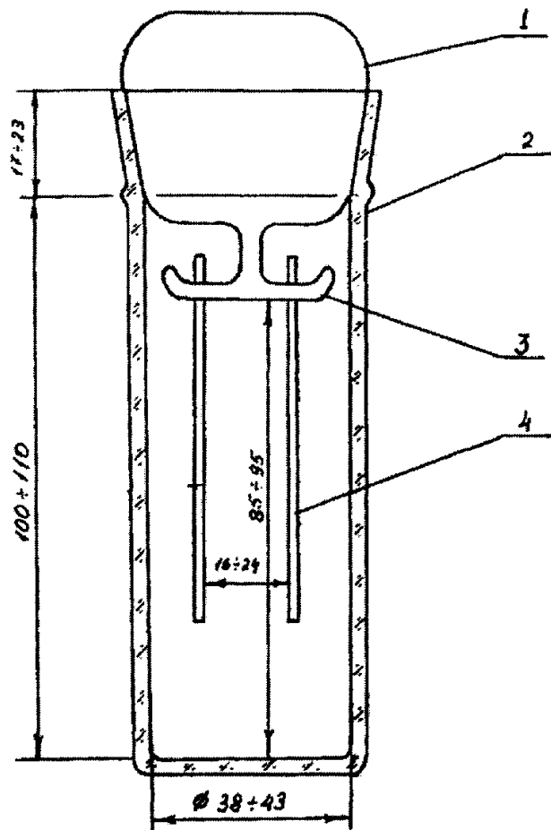
Рисунок 1. Схема лабораторной установки:
